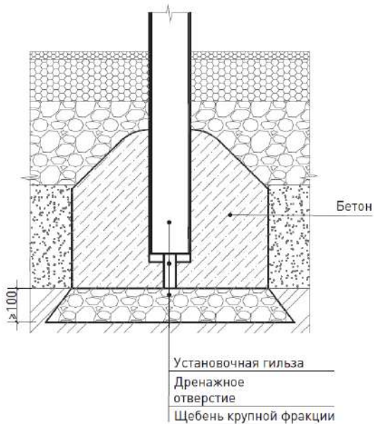
Илл. 3.1.8. СХЕМА МОНТАЖА ИГРОВОГО ОБОРУДОВАНИЯ В ПОКРЫТИЕ ИЗ РЕЗИНОВОЙ КРОШКИ (РЕШЕНИЕ УТОЧНЯЕТСЯ ИНДИВИДУАЛЬНО В ПРОЕКТЕ В ЗАВИСИМОСТИ ОТ МЕСТНЫХ УСЛОВИЙ)
