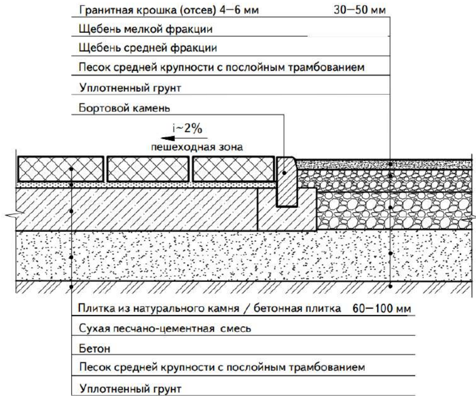
Илл. 1.2.1. ПРИНЦИПАЛЬНАЯ СХЕМА СОПРЯЖЕНИЯ ПЕШЕХОДНОЙ ЗОНЫ ИЗ БЕТОННОЙ ПЛИТКИ (НАТУРАЛЬНОГО КАМНЯ) С ГАЗОНОМ ЧЕРЕЗ БОРТОВОЙ КАМЕНЬ
