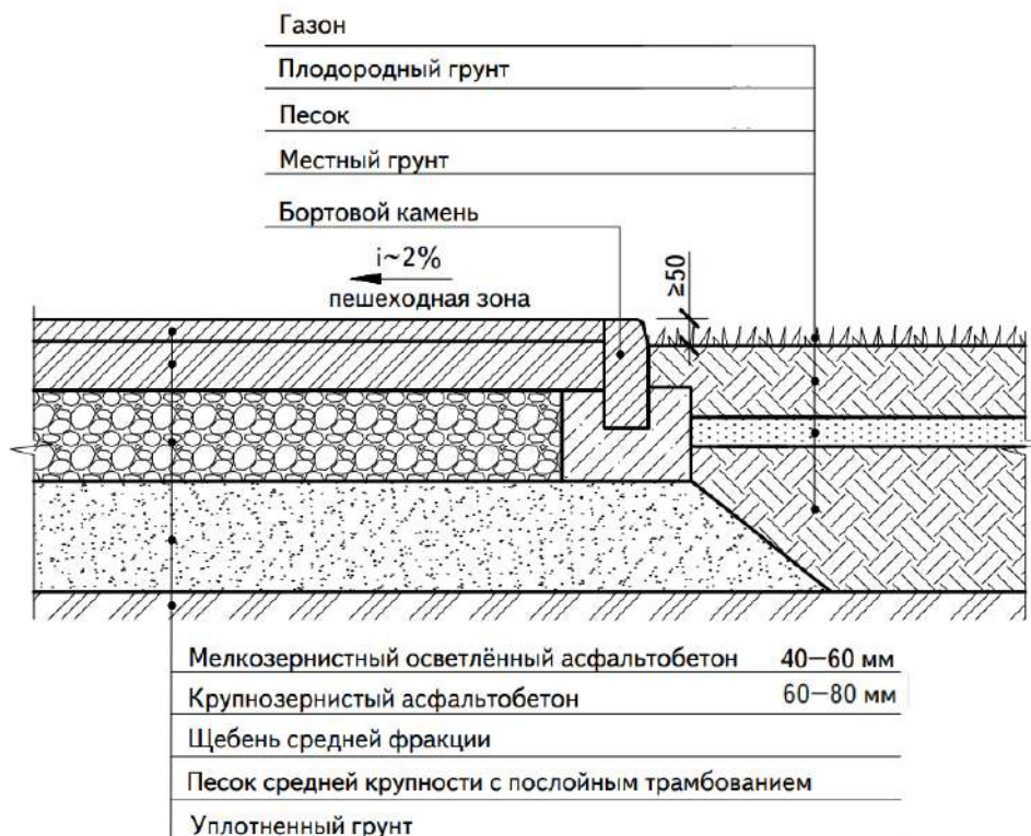
Илл. 1.2.2. ПРИНЦИПАЛЬНАЯ СХЕМА СОПРЯЖЕНИЯ ПЕШЕХОДНОЙ ЗОНЫ ИЗ АСФАЛЬТОБЕТОНА И ГАЗОНА
