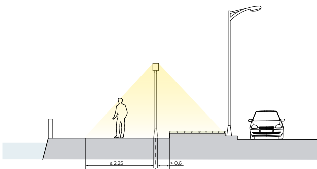
Илл. 1.14 ОДНОСТОРОННЯЯ СХЕМА РАСПОЛОЖЕНИЯ ОПОР ОСВЕЩЕНИЯ
