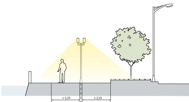
Илл. 1.15 ОСЕВАЯ СХЕМА РАСПОЛОЖЕНИЯ ОПОР ОСВЕЩЕНИЯ
